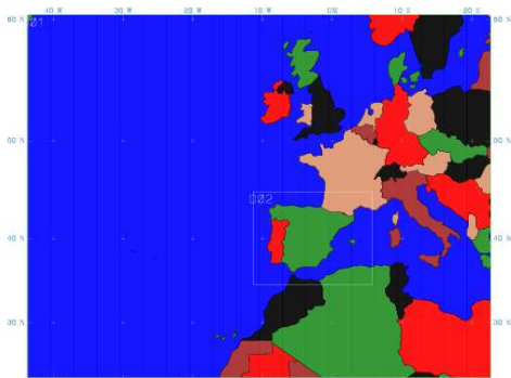
Fig. 3.- Cobertura geográfica de las simulaciones de MM5 para el SPC a corto plazo
