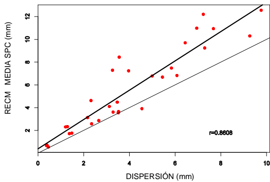
Fig. 5.- Representación de los 31 valores de la dispersión de los miembros respecto a la RECM de la media. El coeficiente de correlación lineal de los mismos es de 0.8608
