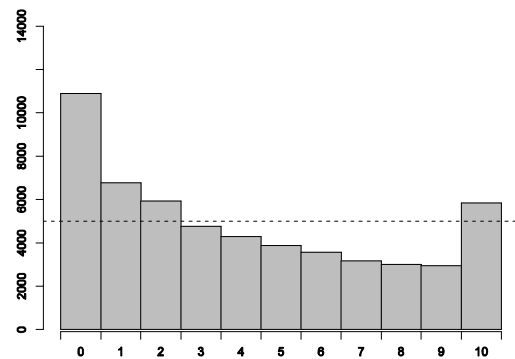
Fig. 6.- Histograma de rangos para la precipitación diaria en el mes de octubre de 2006. La línea en trazo discontinuo indica la equiprobabilidad de los miembros.
