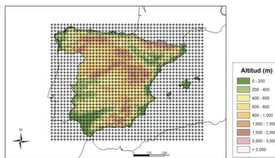
Fig. 2.- Disposición espacial de los puntos en la rejilla de 25 km.
