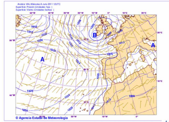
Fig. 13- Presión a nivel del mar (hPa) para el 6 de julio del 2011 a las 12 UTC.
