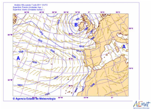
Fig. 14- Presión a nivel del mar (hPa) para el 7 de julio del 2011 a las 12 UTC
