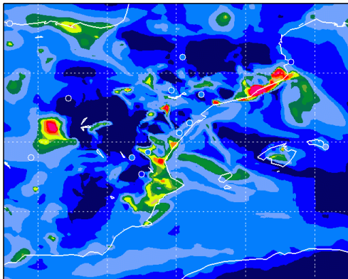
05 Feb 2011 00 UTC AEMET Previsto HH+21 Validado: 05 Feb 2011 21 UTC Modelo: MOCAGE MACCH3 Altura: Superficie Parametro: NO_2 [ug/m3]
