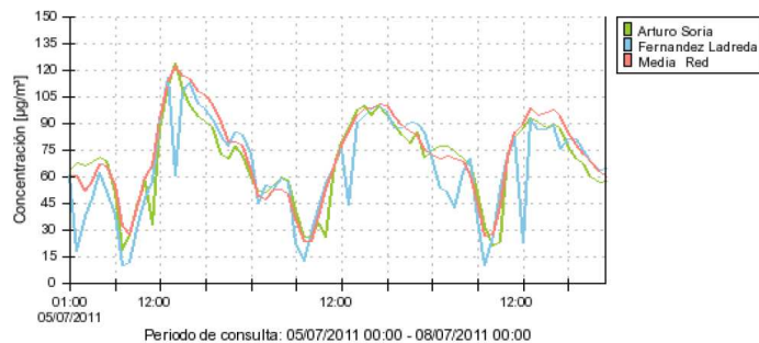
Fig. 18.- Concentración de O 3 (µg/m 3 ) en promedio horario en las estaciones de calidad del aire madrileñas entre los días 5 de julio del 2011 y 7 de julio del 2011
