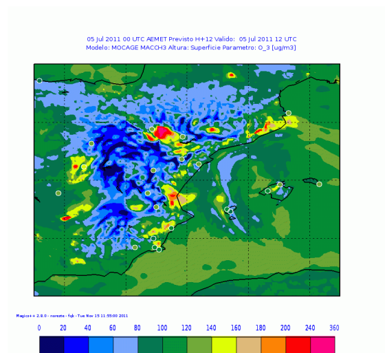
Fig. 15.- Predicción de concentración de O 3 (µg/m 3 ) con MACCH3 MOCAGE planteando las observaciones de la red de estaciones para el 5 julio de 2011 a la hora 12:00 UTC.
