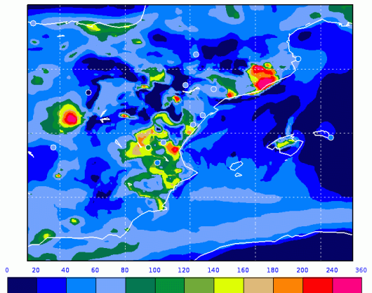
07 Feb 2011 00 UTC AEMET Previsto HH+21 Validado: 07 Feb 2011 21 UTC Modelo: MOCAGE MACCH3 Altura: Superficie Parametro: NO_2 [ug/m3]
