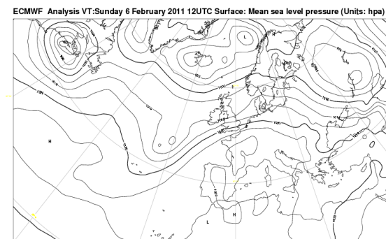
Fig. 4.- Presión a nivel del mar (hPa) para el 6 de febrero del 2011 a las 12 UTC.
