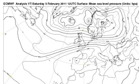
Fig. 3.- Presión a nivel del mar (hPa) para el 5 de febrero del 2011 a las 12 UTC.
