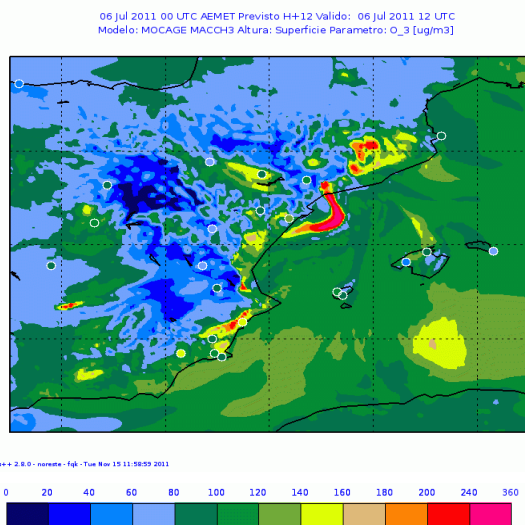
Fig. 16.- Predicción de concentración de O 3 (µg/m 3 ) con MACCH3 MOCAGE plotando las observaciones de la red de estaciones para el 6 julio de 2011 a la hora 12:00 UTC.
