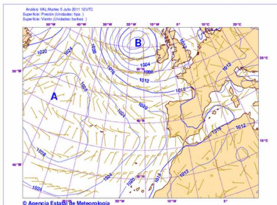
Fig. 12- Presión a nivel del mar (hPa) para el 5 de julio del 2011 a las 12 UTC.
