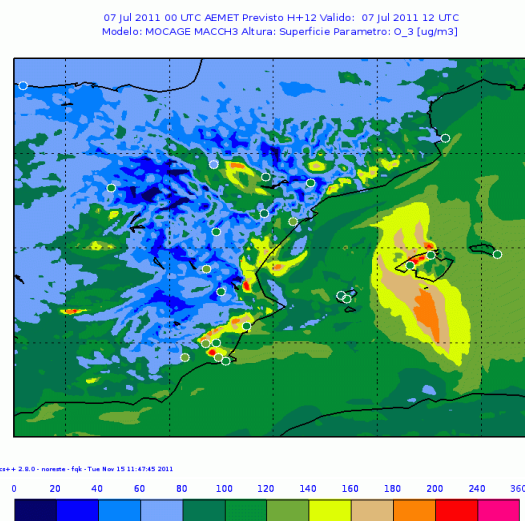
Fig. 17.- Predicción de concentración de O 3 (µg/m 3 ) con MACCH3 MOCAGE plotando las observaciones de la red de estaciones para el 7 julio de 2011 a la hora 12:00 UTC.
